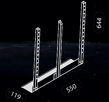
Standard 12 cm - Holme verlängert 550 x 119 x 644 mm
