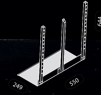
25 cm - Holme verlängert 550 x 249 x 644 mm
